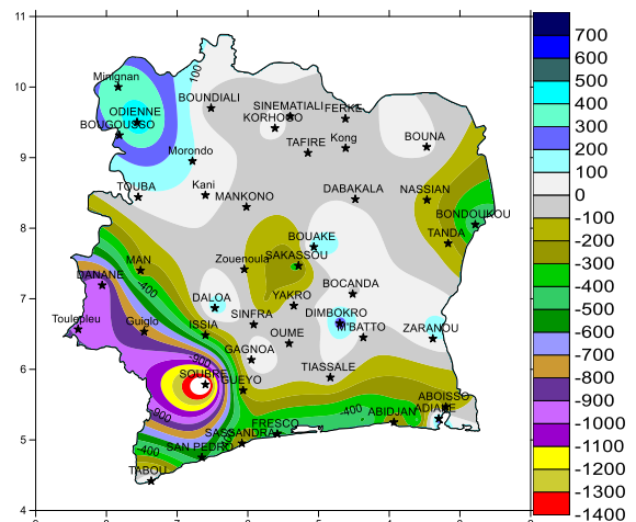
Fig. 4 : Ecart entre Cumuls pluviométriques du 1 Janvier au 20 Novembre 2019 et du 1 Janvier au 20 Novembre de la normale (1981-2010)
