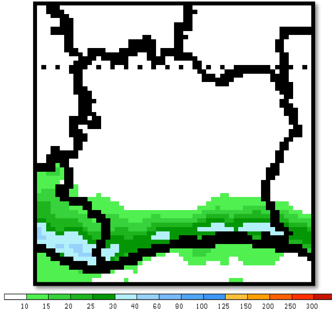
Fig.10: prévision de la pluviométrie du 26 Novembre au 03 Décembre. 2019 (source : NOAA, climat Prédiction Center)
