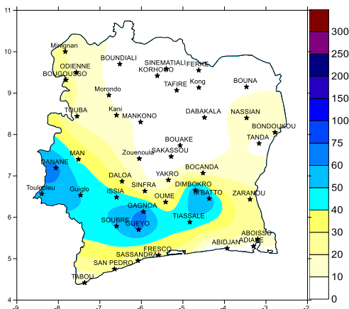
Fig1 : Pluviométrie totale (mm) du 11 au 20 Novembre 2019
