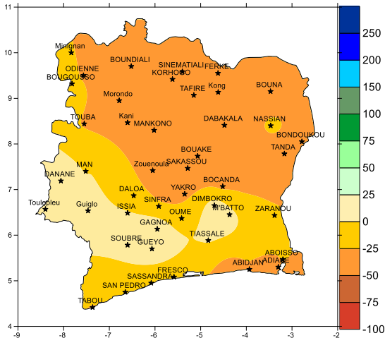
Fig. 9 : Bilan hydrique climatique (mm) du 11 au 20 Novembre 2019
