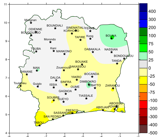
Fig2 : Ecart entre la pluviométrie (mm) du 11 au 20 Novembre 2019 et du 11 au 20 Novembre de la normale
