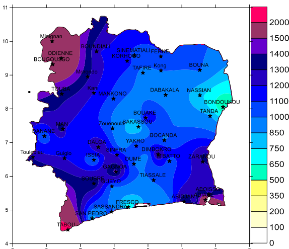
Fig. 3 : Cumul pluviométrique (mm) du 11 Janvier au 20 Novembre 2019
